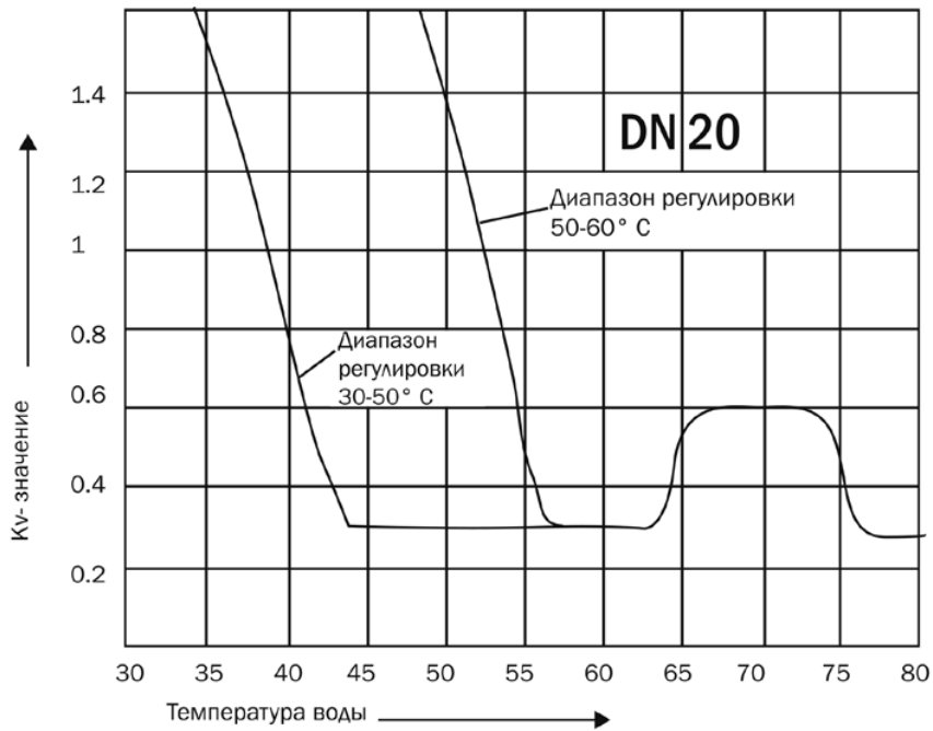
Характеристика DN20 диапазон регулировки 50-60° C
