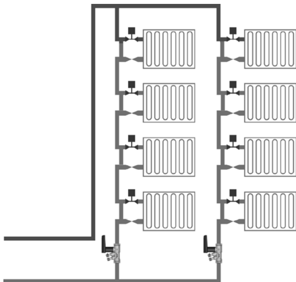
Однотрубная система отопления (Heizen Smart)
