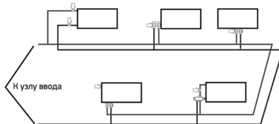
Коллекторно лучевая, периметральная схема систем отопления
