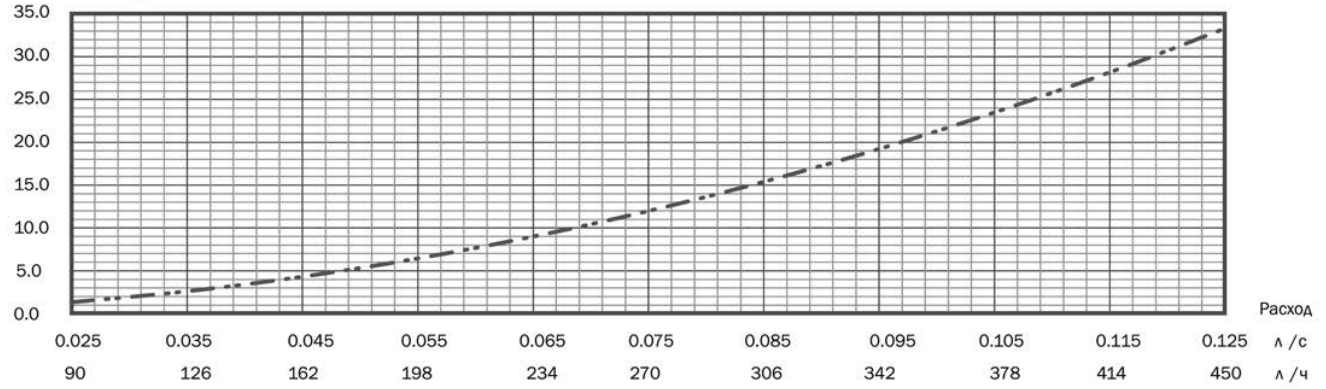
График перепада давления на измерительных ниппелях от расхода
