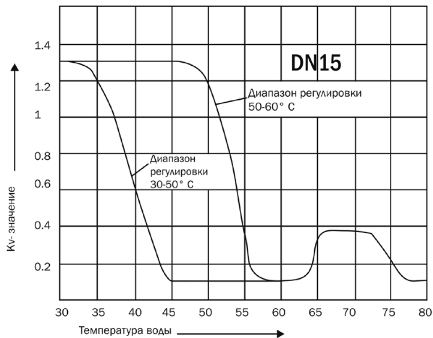
Характеристика DN15 диапазон регулировки 50-60 ° C
