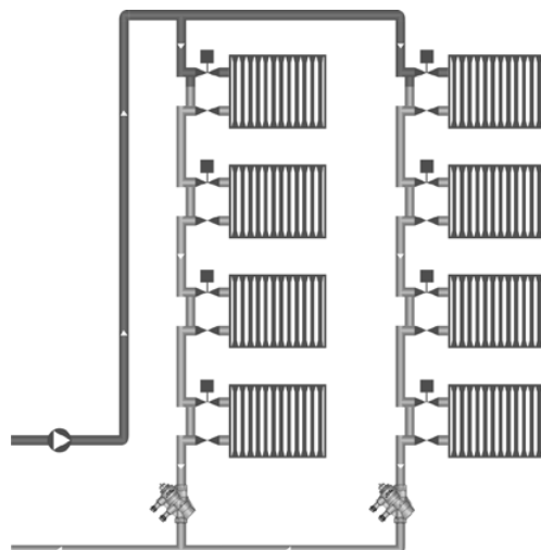
Автоматическая балансировка на однотрубной системе отопления (Heizen Control)
