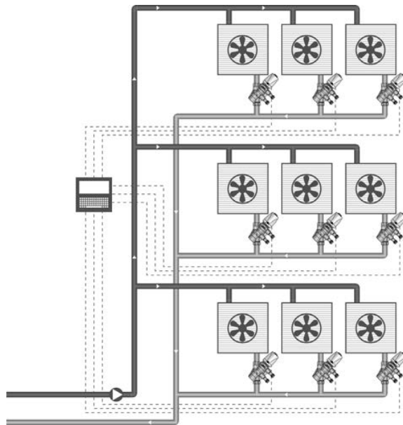
Балансировка на ветви фэнкойлов (Heizen Control)
