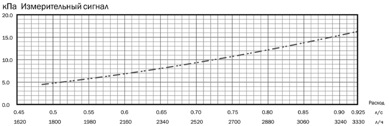
График перепада давления на измерительных ниппелях от расхода
