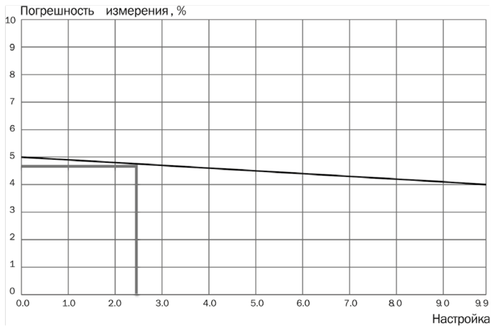
Зависимость погрешности измерения от настройки клапана
