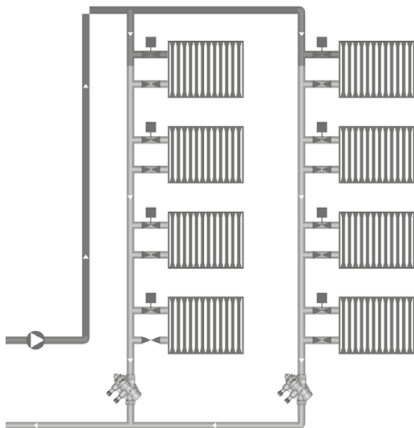
Пример 1. Балансировка стояков однотрубной стояковой системы с термoelementами.
