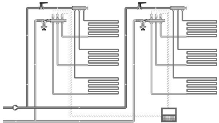
Балансировка перед коллектором системы внутриспольного отопления (Heizen Auto+ Heizen Lock)
