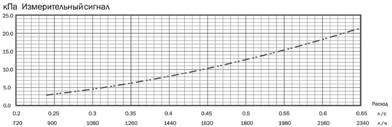
График перепада давления на измерительных ниппелях от расхода
