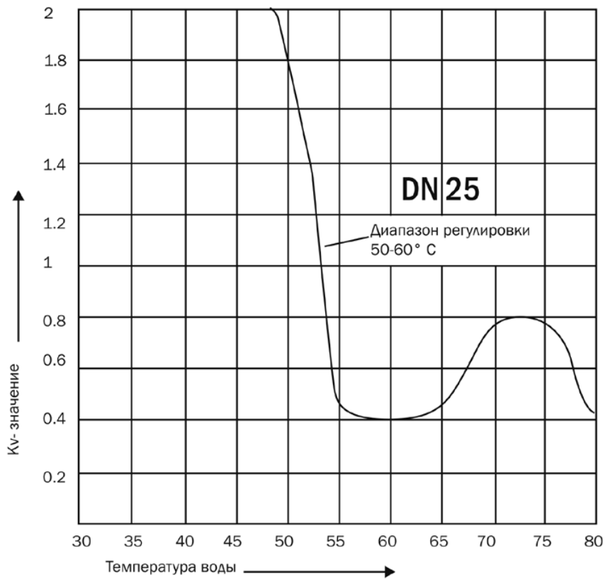
Характеристика DN25 диапазон регулировки 50-60° C
