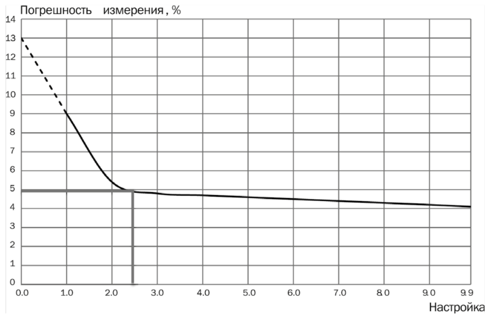
Зависимость погрешности измерения от настройки клапана
